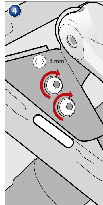
Maniglia Sollevamento Moto BMW F800R/S/ST Codice 20530-102
