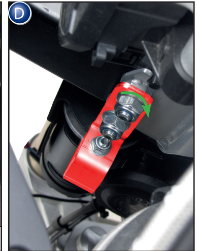
Neue Schrauben / new screws
